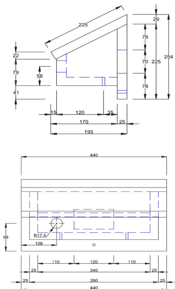
slika 2: mere StoElement Fauna SP-F 20
