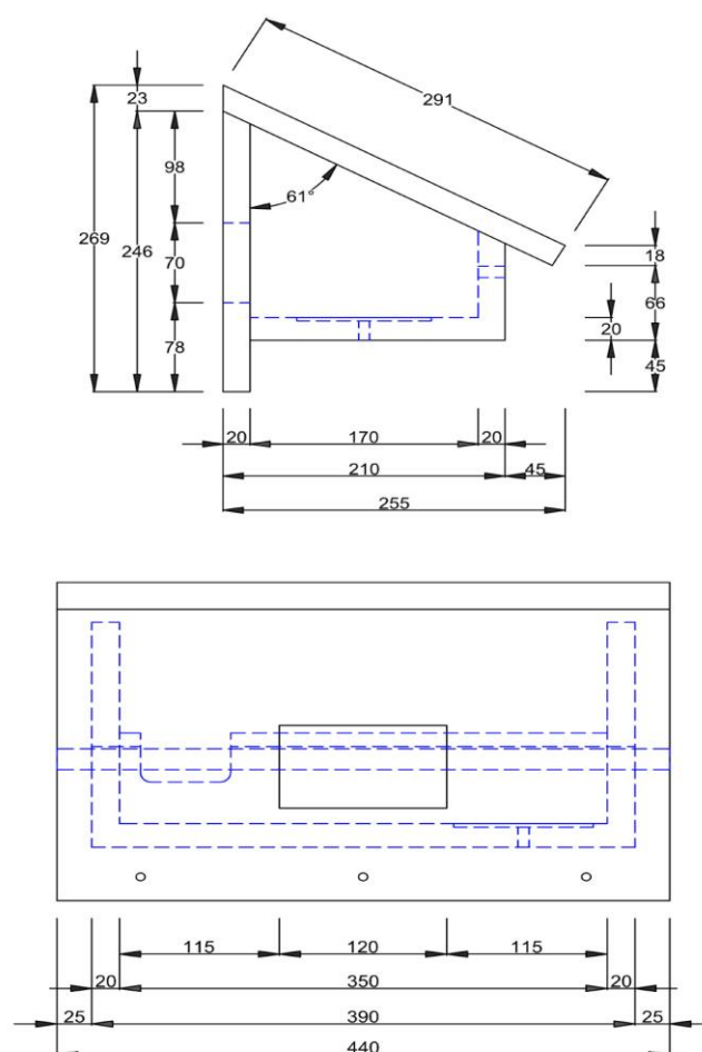
slika 2: mere StoElement Fauna MS-F 20
