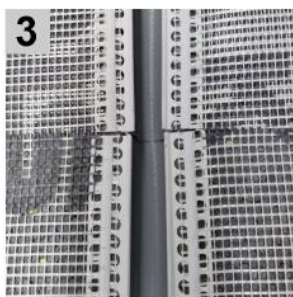
oblikovanje spojev pri izdelku Sto-Dehnfugenprofil E
