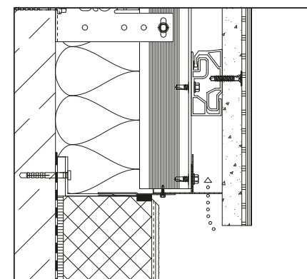
Vertikalschnitt Sockelanschluss
