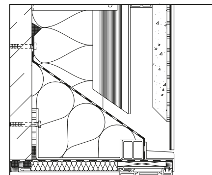
Vertikalschnitt
