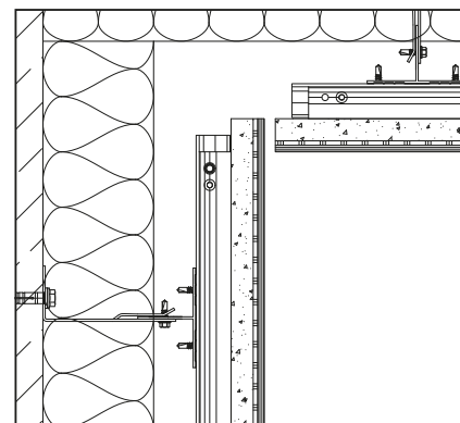
Horizontalschnitt Innenecke mit Überstand
