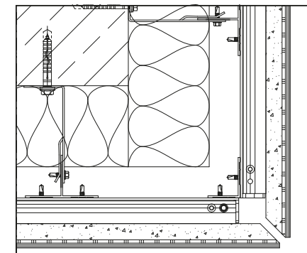
Horizontalschnitt Außenecke auf Gehung
